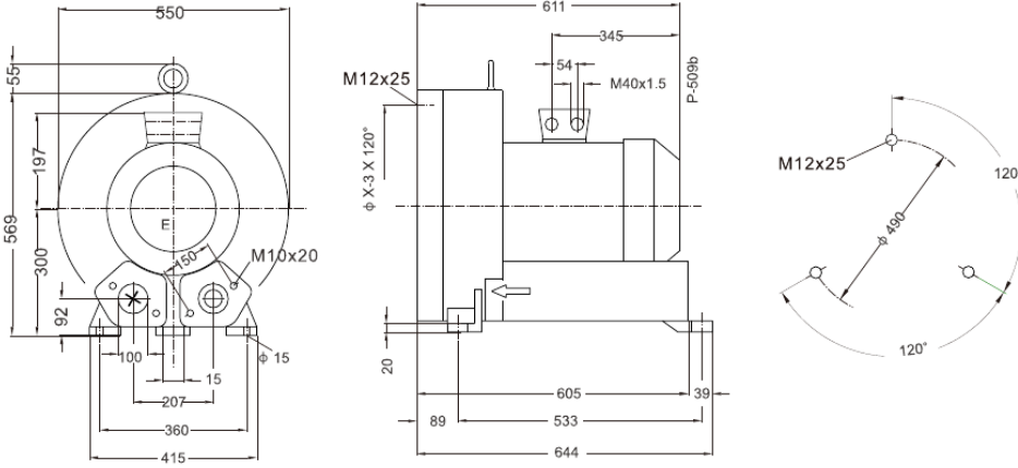
Montaj ve Ölçüler (mm)
