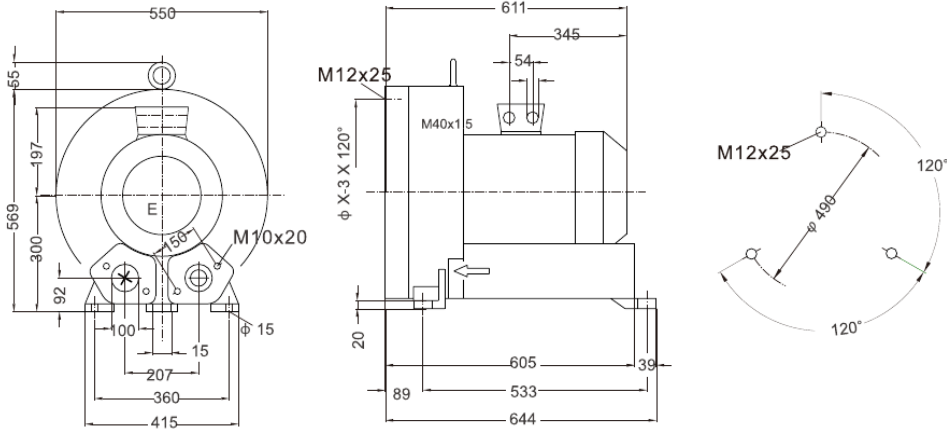
Montaj ve Ölçüler (mm)
