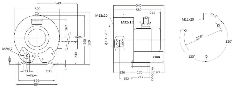
Montaj / Ölçü Şeması (mm)
