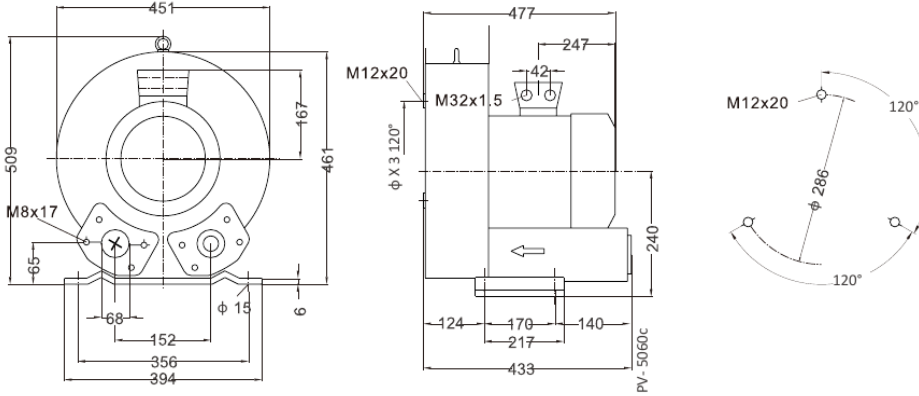
Montaj ve Ölçüler (mm)
