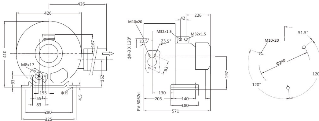
Montaj / Ölçü Şeması (mm)
