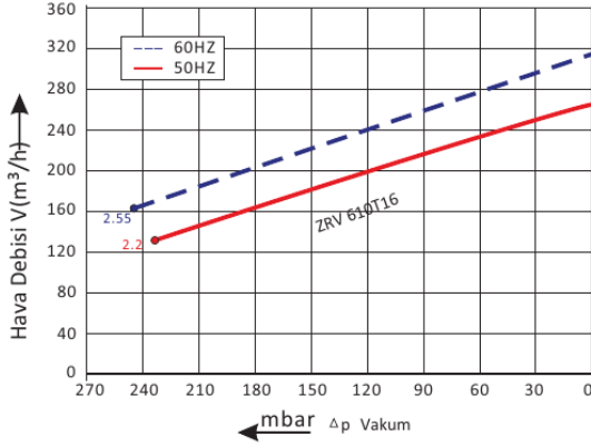
Vakum Performans Eğrisi
