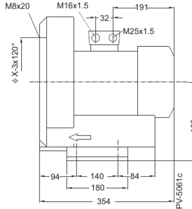
Montaj ve Ölçüler (mm)
