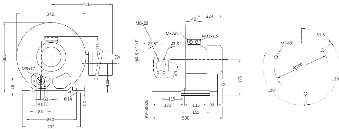
Montaj / Ölçü Şeması (mm)
