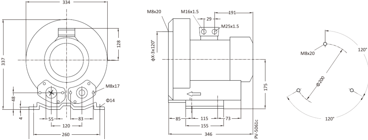
Montaj ve Ölçüler (mm)
