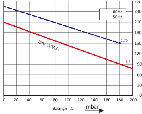
Basınç Performans Eğrisi
