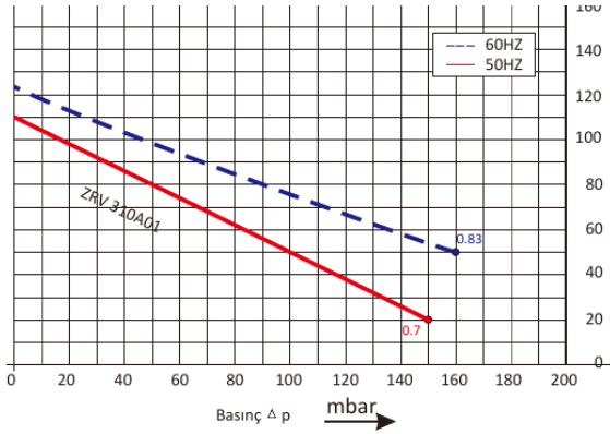
Basınç Performans Eğrisi
