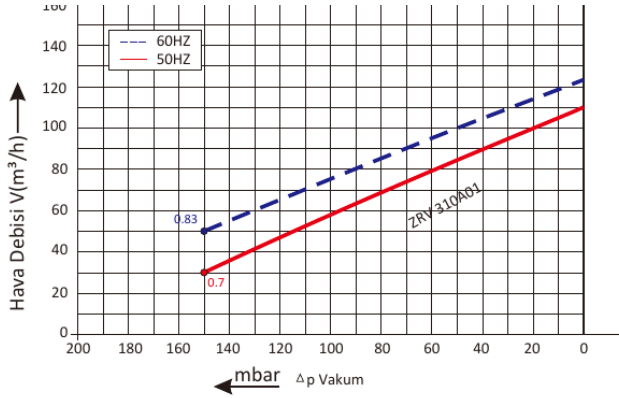
Vakum Performans Eğrisi
